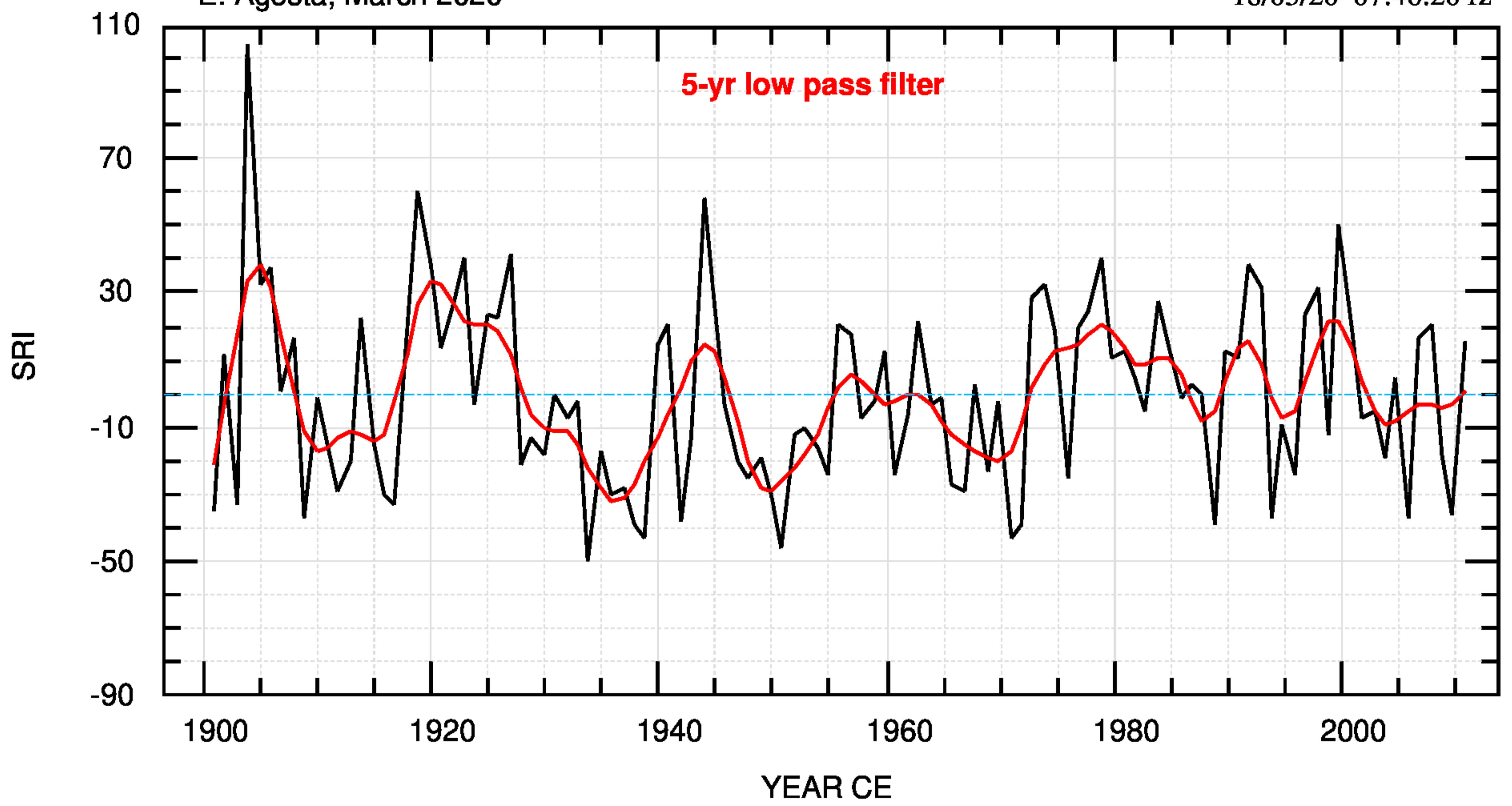
agosta.txt
