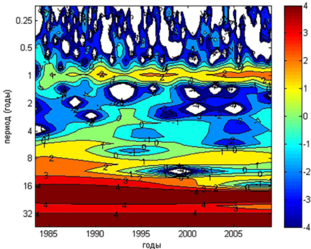
Рис. 5. Вейвлет-анализ ряда глобальной общей облачности по данным ISCCP (значения спектральной плотности).
